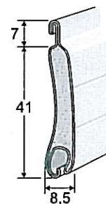
Lamellprofil HR41 ECO
