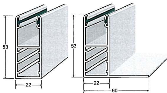
Styrskena HTF och L-HTF 1
