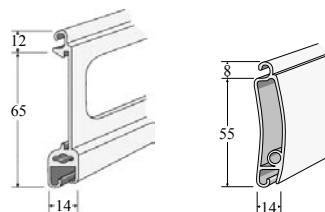
Lamellprofil GR 6502 och VST 5110
