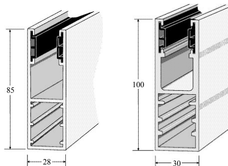
Styrskena H-STF och SH-STF
